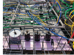
안산 메트로푸르지오힐스테이트 기계설비공사 연천군 은대지구 공동주택 기계설비공사 급배수 위생배관 / SR-JOINT 이중관 소방배관 / C-PVC
