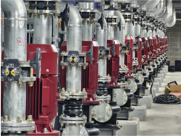
김해안동 쿠팡 스마트물류센터 UNIT COOLER 66 SET SCREW 냉동기 15 SET 냉각탑 500RT 4 SET
